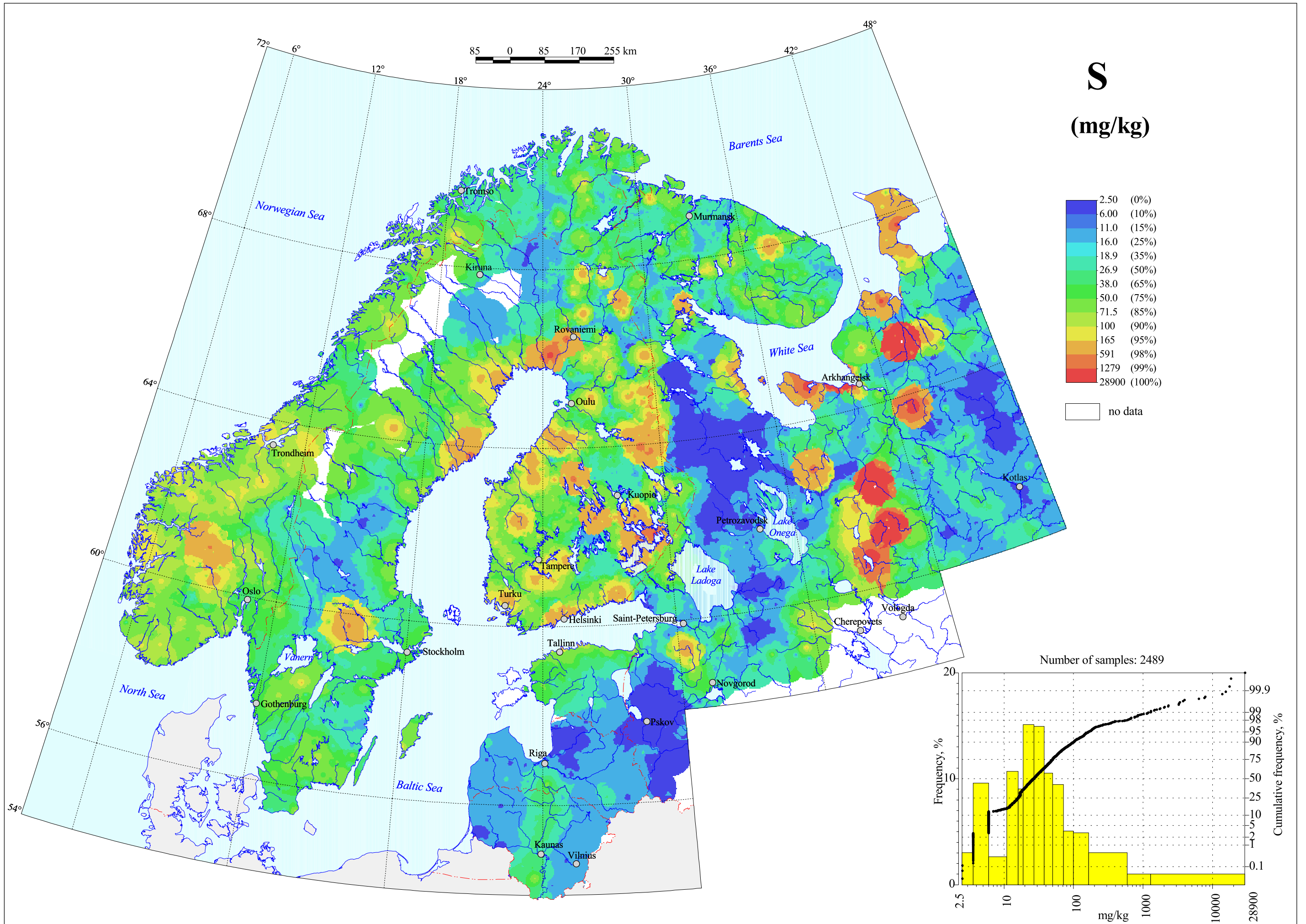
Sulphur in C-horizon, Grain Size <2 mm, Aqua regia Extraction
